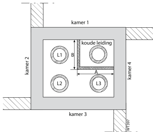
Afb. 3.7 Doorsnede leidingschacht
