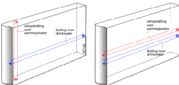
Afb. 4.8 Waterleiding in wand achter radiator (niet toegestaan)
