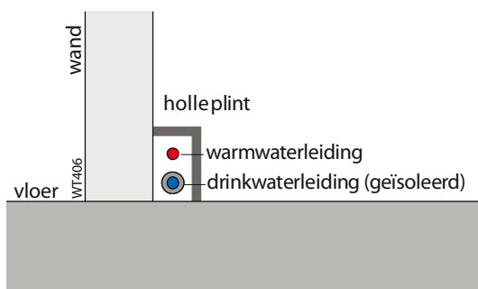
Afb. 3.6 Leiding voor drinkwater en een uittapleiding voor warm tapwater weggewerkt in een holle plint of achter een voorzetwandsysteem
