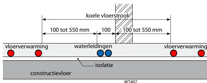
Afb. 4.1 Een 'koele vloerstrook' bij een vloer met tussenisolatie
