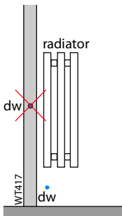
Afb. 4.8 Waterleiding in wand achter radiator (niet toegestaan)
