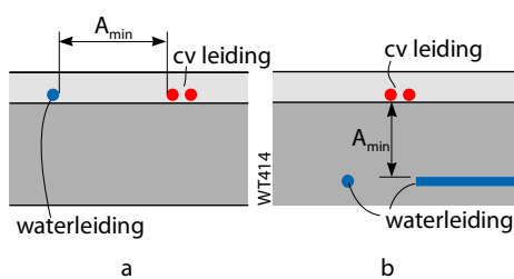
Afb. 4.4 Minimum afstanden A_{min} tussen waterleiding en CV-leidingen en/of circulatieleidingen voor warmtapwater in tabel 4.1
