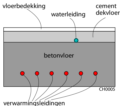
Afb. 5.1 Waterleiding in cement dekvloer op een vloer met betonkernactivering (28 °C).
