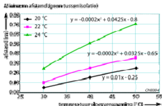
Afb. 4.13 Interpolatie bij andere aanvoertemperaturen vloerverwarming
