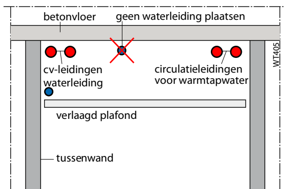
Afb. 3.5 Waterleiding laag boven verlaagd plafond (CV- en circulatieleidingen voldoende isoleren)
