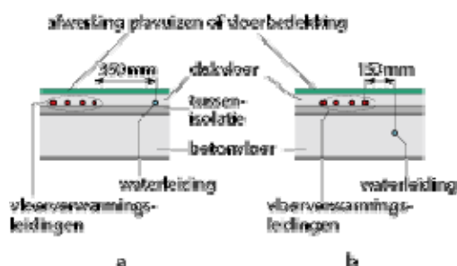
Afb. 4.11 Minimum afstanden van voorbeeld 4
