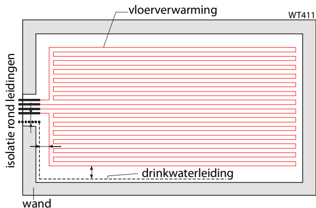
Afb. 4.14 Waterleiding in vloer met vloerverwarming; Toegestaan mits op minimum afstand in tabel 4.3 en 4.4, kolom nr. 6 en 7.
