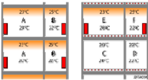
Afb. 4.2 Temperaturen en temperatuurgelaagdheid in ruimten met radiator- en met vloerverwarming (De coderingen A t/m F worden toegepast in tabellen 4.1, 4.3 en 4.4)
