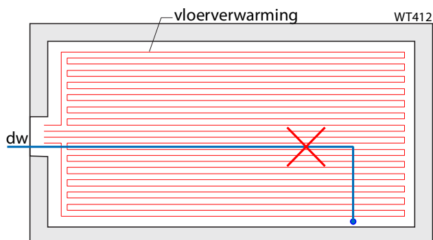
Afb. 4.15 Waterleiding kruist vloerverwarming; Soms toegestaan, zie tabel 4.3 en 4.4, kolom nr. 7.
