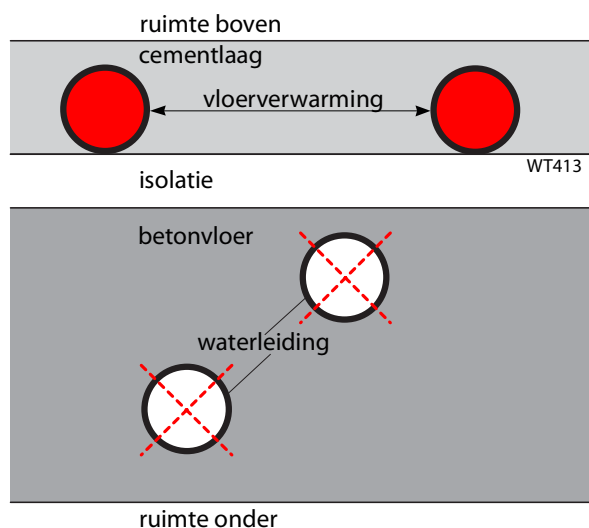
Afb. 4.16 Waterleiding kruist vloerverwarming onder isolatie; Soms toegestaan, zie tabel 4.3, kolom nr.7
