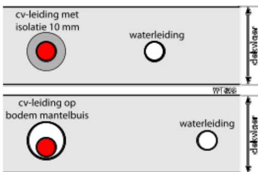
Afb. 4.3 De minimum afstand is mede afhankelijk van isolatie van de warme leiding
