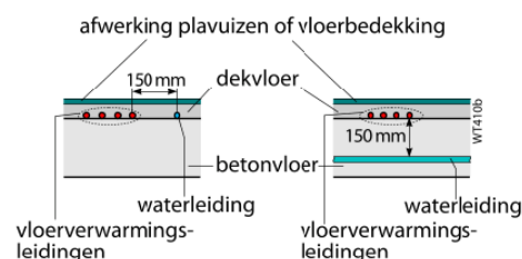
Afb.4.12 Minimumafstanden van voorbeeld 5
