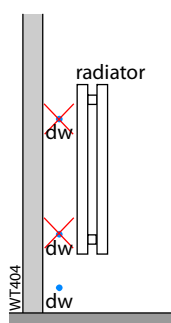
Afb. 3.4 Waterleiding achter radiator
