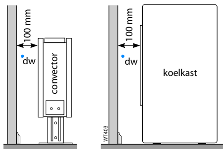
Afb. 3.3 Waterleiding achter koelapparaat of convector
