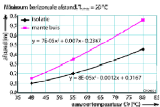
Afb. 4.5 Interpolatie bij andere CV-aanvoertemperaturen
