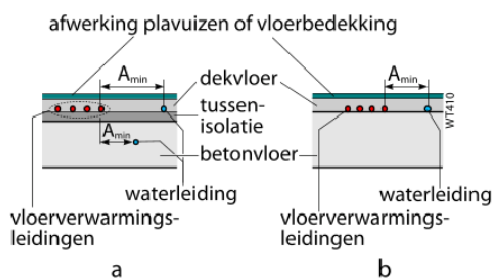
Afb. 4.10 Minimum afstanden A_{min} vanaf vloerverwarmingsleidingen in tabel 4.3 en 4.4
