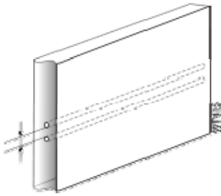
Afb. 4.6 Waterleiding en warme leiding (CV-leidingen of circulatieleidingen voor warmtapwater) in wand evenwijdig aan elkaar
